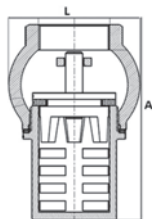
ART. TT687 Válvula Artesiana Extremos rosca GAS ISO 228/1 Veio em balão Max temp.: 110°C
