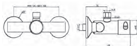
ART.08132 Misturadora Chuveiro Temporizada
