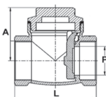
ART. TT314 Válvula c/ Postigo Vedação Borracha Extremos rosca GAS ISO 228/1 Pressão abertura: 0,03bar Max temp.: 110°C Montagem horizontal
