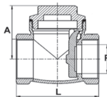
ART. TT313 Válvula c/ Postigo Vedação Metal Extremos rosca GAS ISO 228/1 Pressão abertura: 0,03bar Max temp.: 110°C Montagem horizontal
