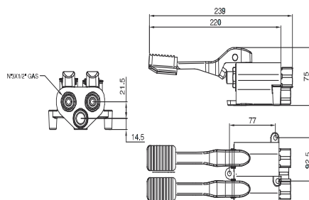
ART.02066 Misturadora 2 Pedais Horizontal
