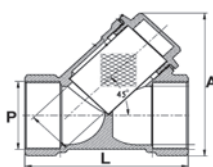
ART. TT319 Filtro impurezas Tipo Y Extremos rosca GAS ISO 228/1 Filtro em Aço inox Max temp.: 110°C
