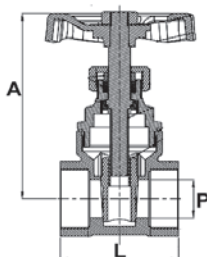
ART. TT304 Passador Adufa Composição em latão Passagem total Extremos rosca GAS ISO 228/1 Max temp.: 100°C
