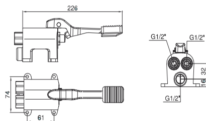
ART.02070 Misturadora Pedal Horizontal
